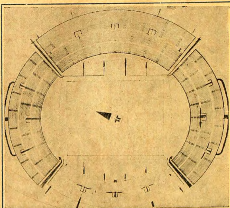
La planta del estadio. La cancha y las instalaciones detalladas. Se puede ver, en el centro, el estadio, y los pequeños círculos. En reducida escala indican ellos las boleterías que servirán para las localidades populares.
