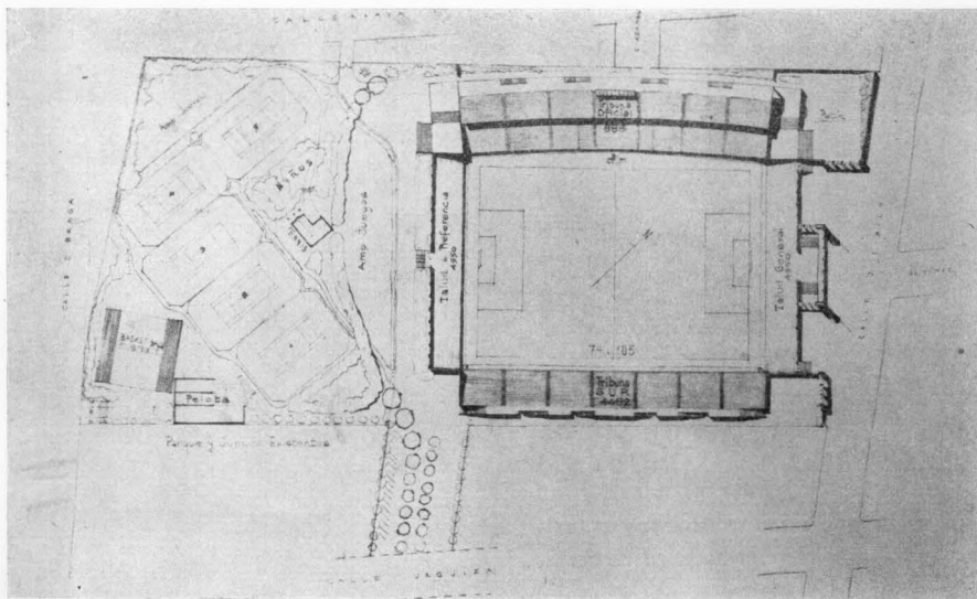
Planta general
