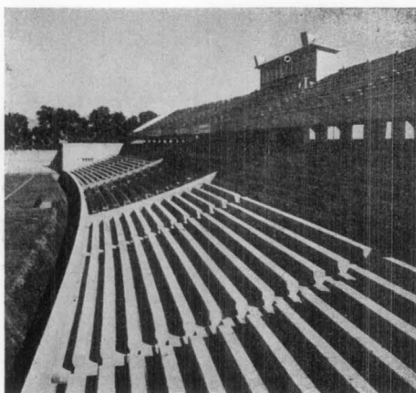
Graderías
