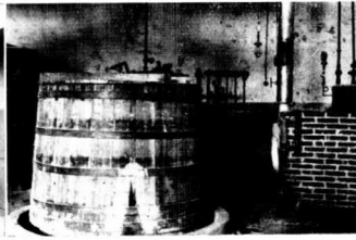
TINA DE CATALIZACION Y DESDOBLAMIENTO
