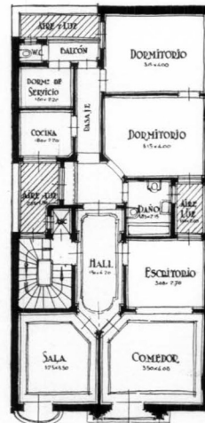
PLANTAS ALTAS
