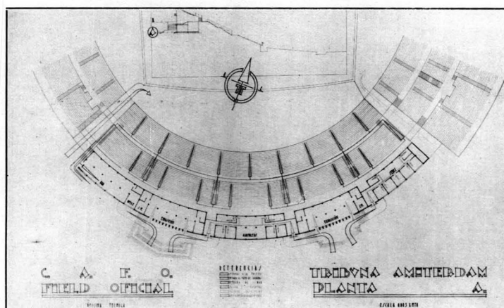
Planta baja de la tribuna Amsterdam
