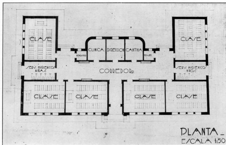
PLANTA
