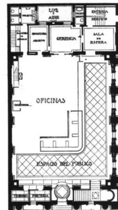
Planta baja
