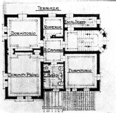
Planta alta
