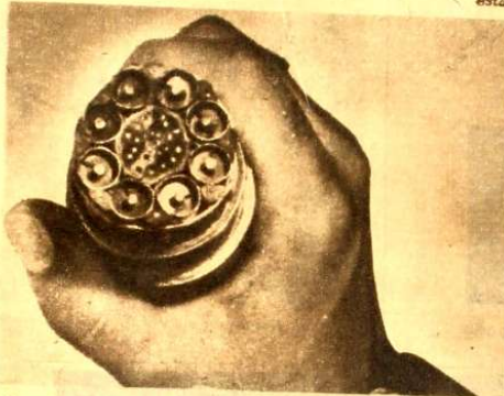
Sección normal de un cable coaxial de ocho cables, que es la base de uno de los sistemas de transmitir televisión. No puede transmitirse televisión por el simple cable telefónico, como se realiza con radio.
